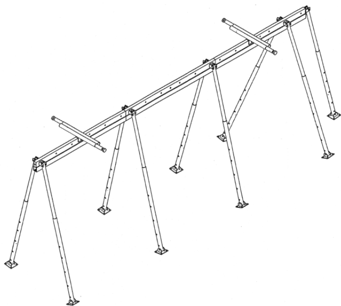
Schéma du portique (3 modules de 2 m) (déjà présenté dans LSB Info n°48 – Robert Rouvidant)
